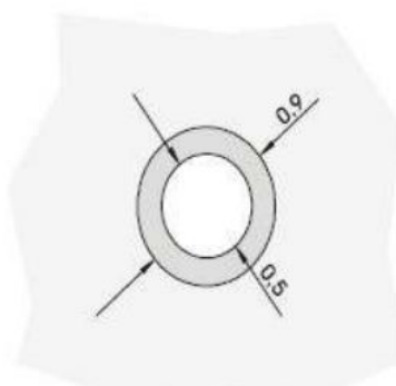
Figura 7 - Detalhes do ilhós
