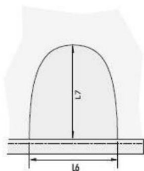
Figura 6 - Detalhes da aba de sustentação da boina
