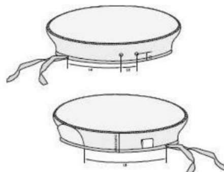
Figura 8 - Detalhes de fixação do ilhós na boina
